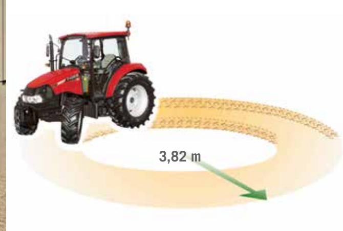
Rayon de braquage de 3,82 m (Farmall 55 C - 75 C) et de 4,33 m (Farmall 85 C - 115 C).
