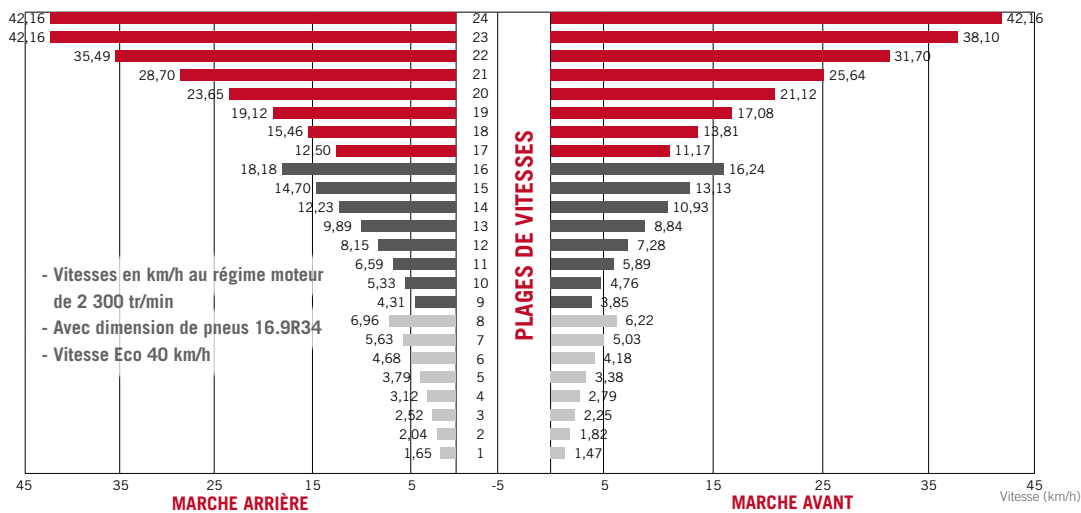
Schéma de vitesses de la transmission 24x24 Hi Lo 40 km/h
